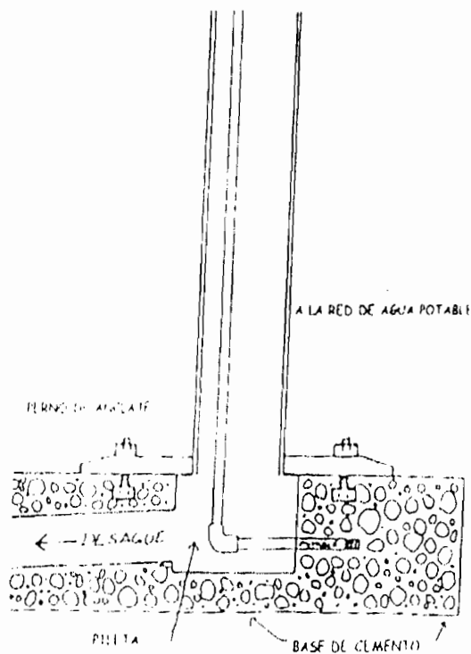
INSTALACION BASICA
